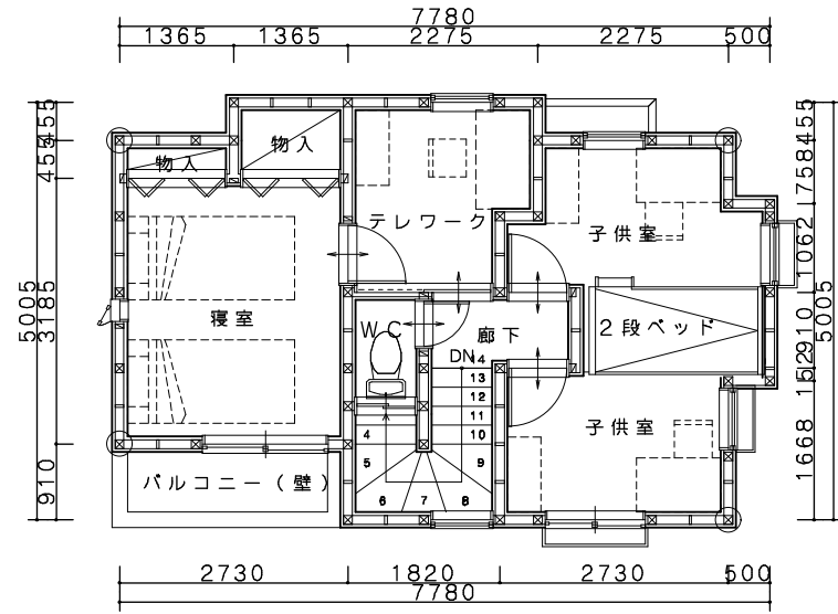
2階平面図
