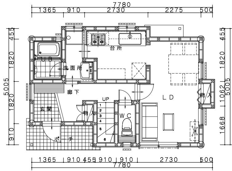
1階平面図
