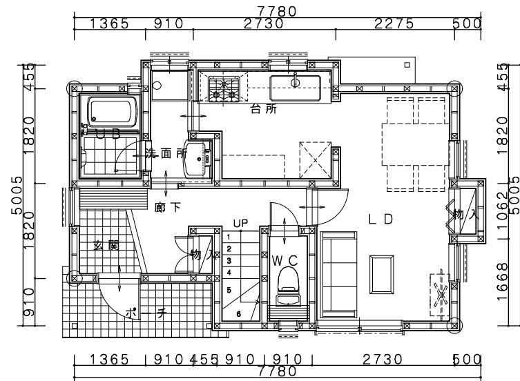
1階平面図
