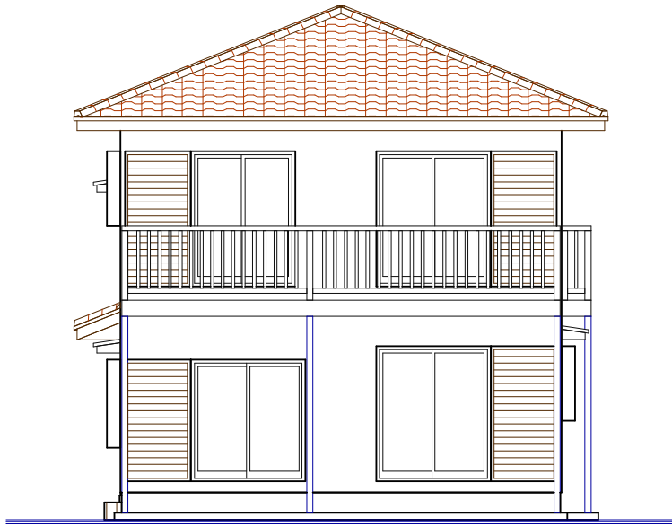
南側立面図
