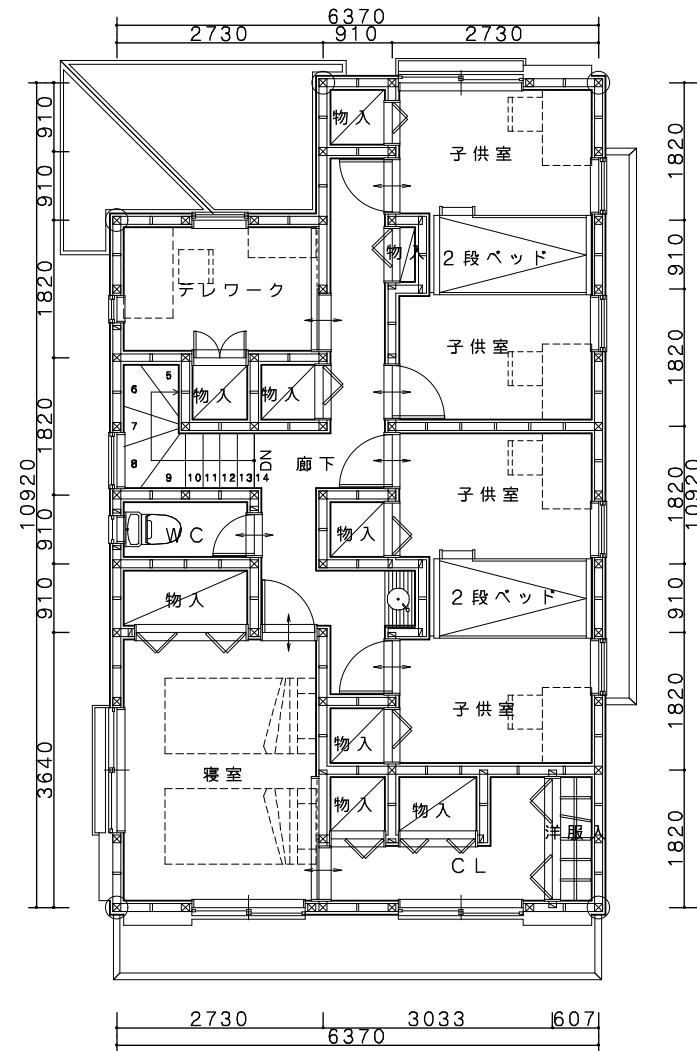
2階平面図
