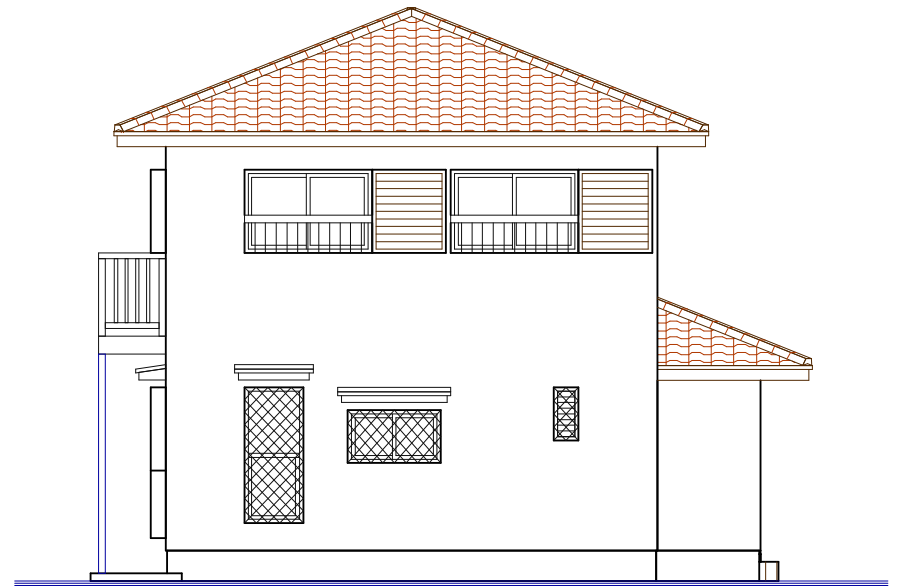
東側立面図
