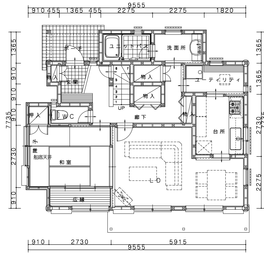
1階平面図
