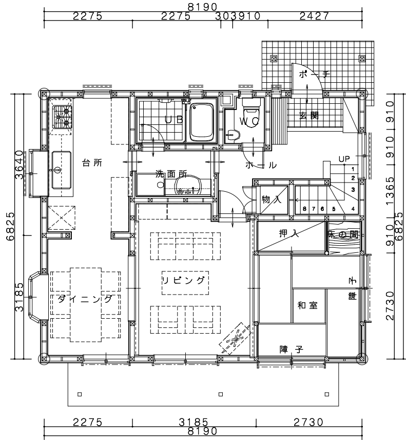
1階平面図
