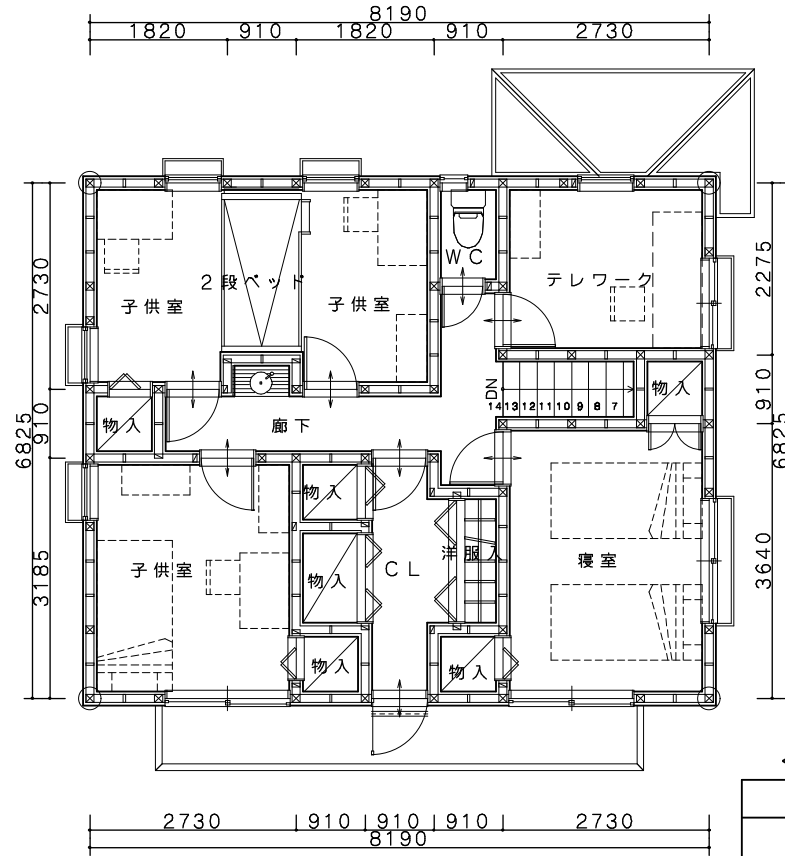
2階平面図
