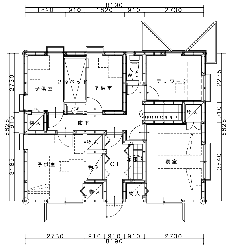
2階平面図
