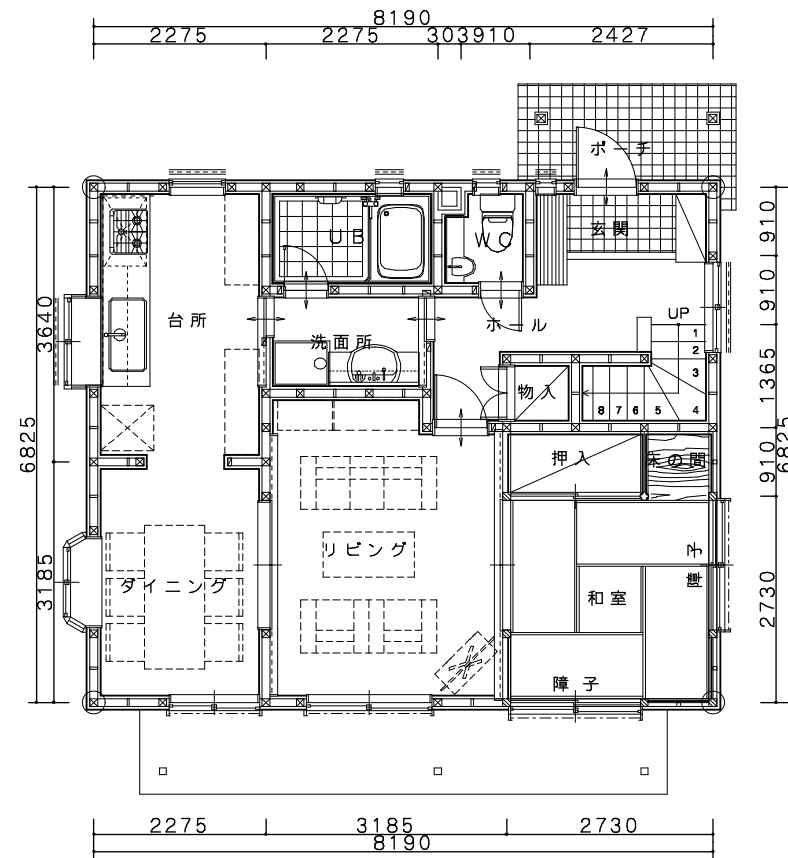
1階平面図
