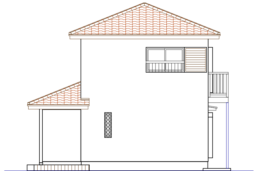
西側立面図
