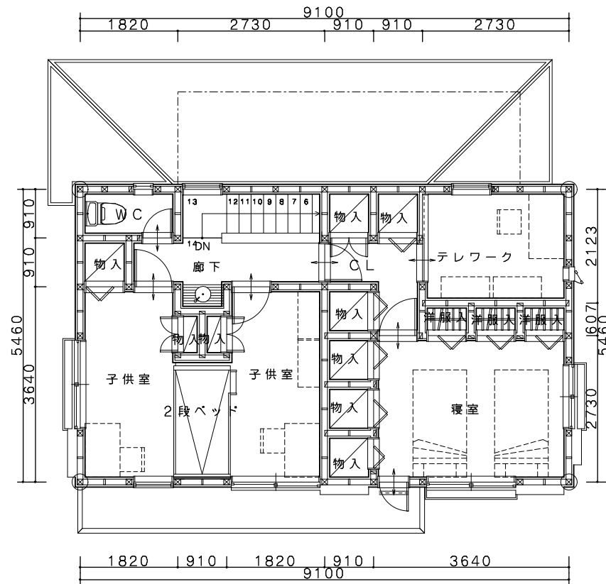
2階平面図
