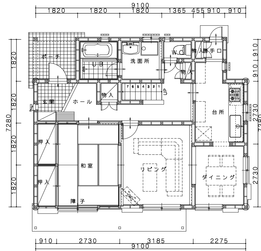
1階平面図
