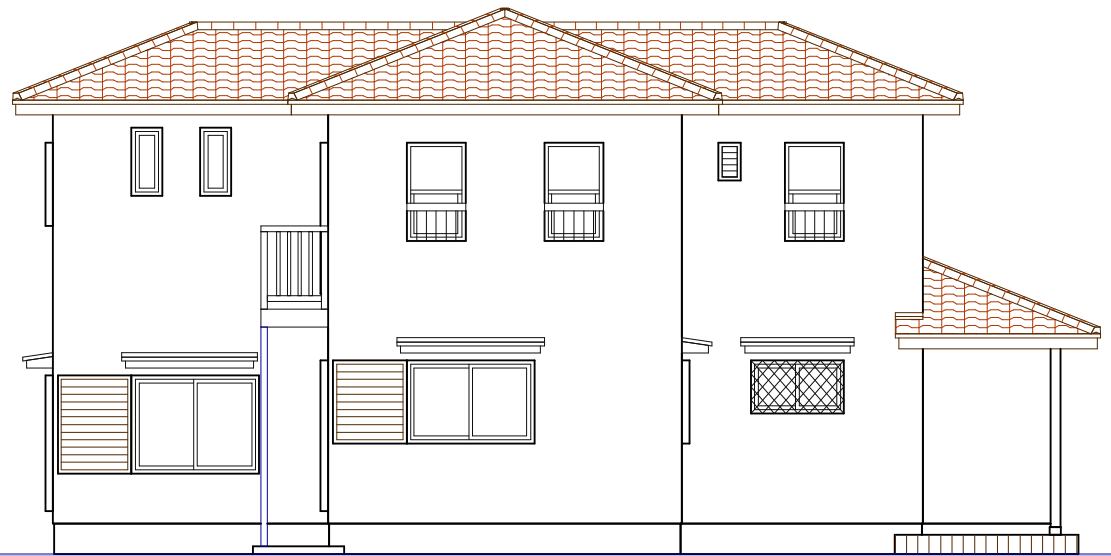
東側立面図
