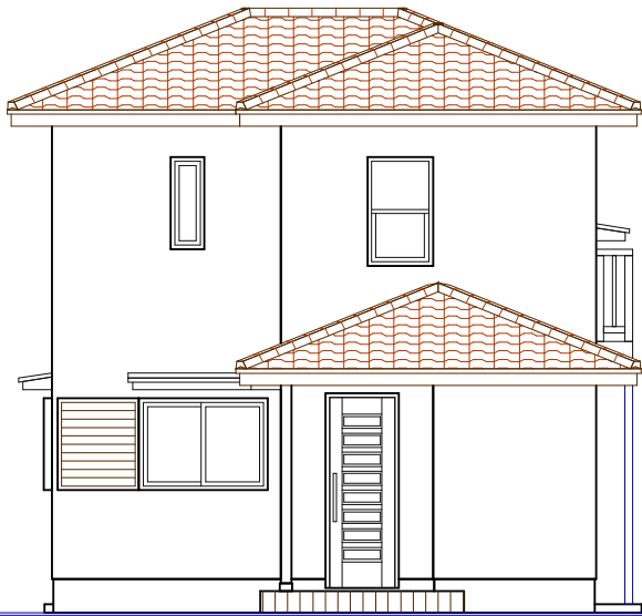
北側立面図
