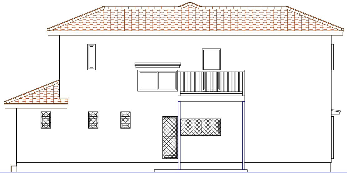
西側立面図
