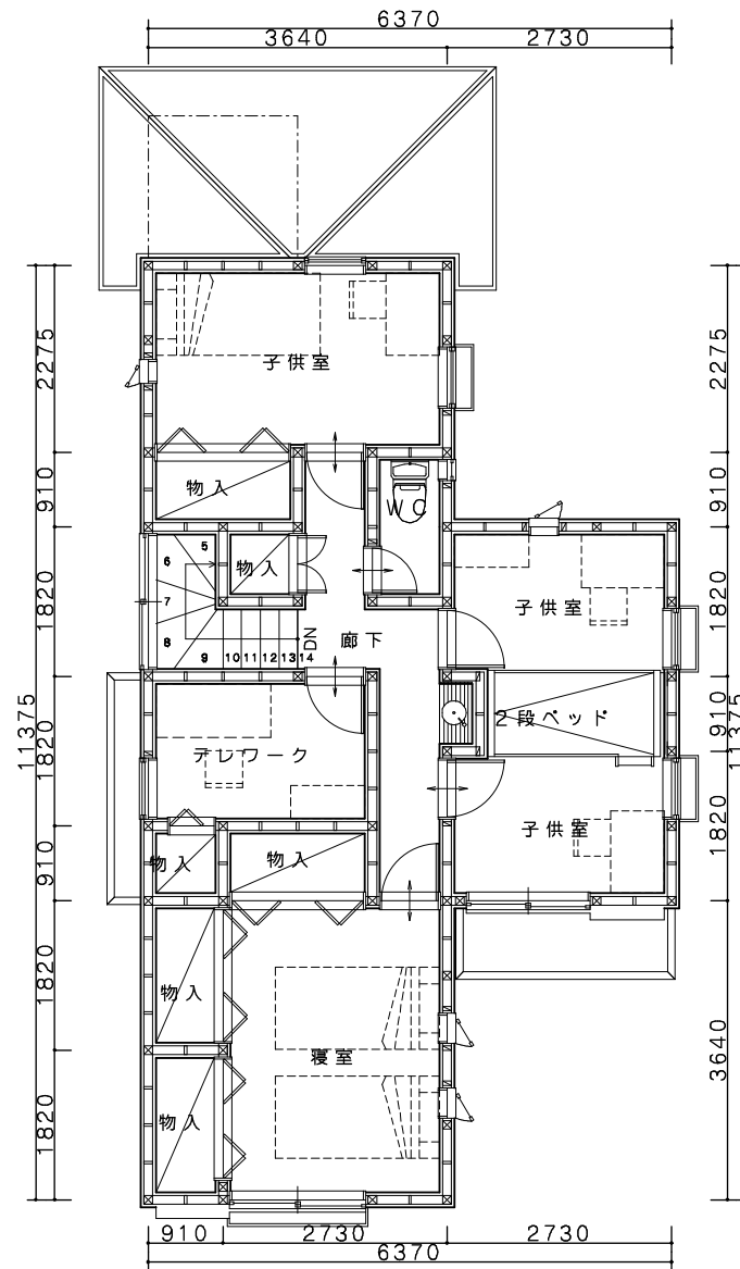
2階平面図
