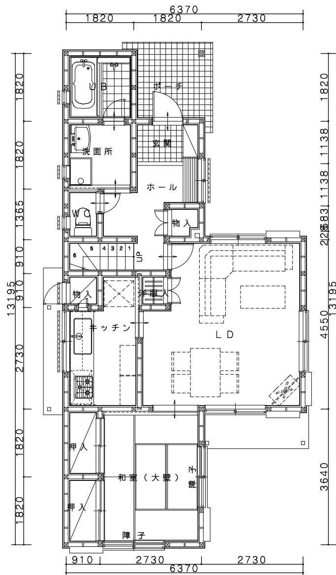
1階平面図
