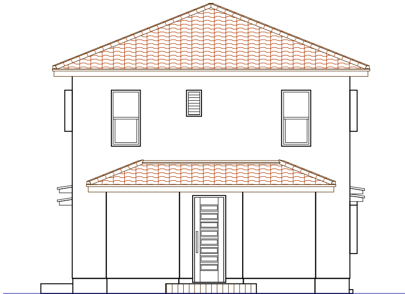
北側立面図
