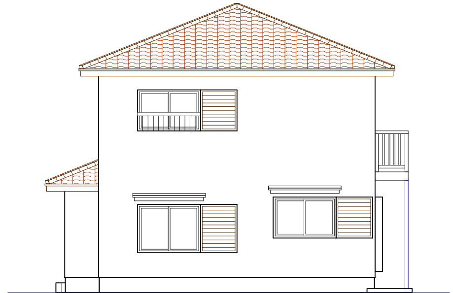
西側立面図
