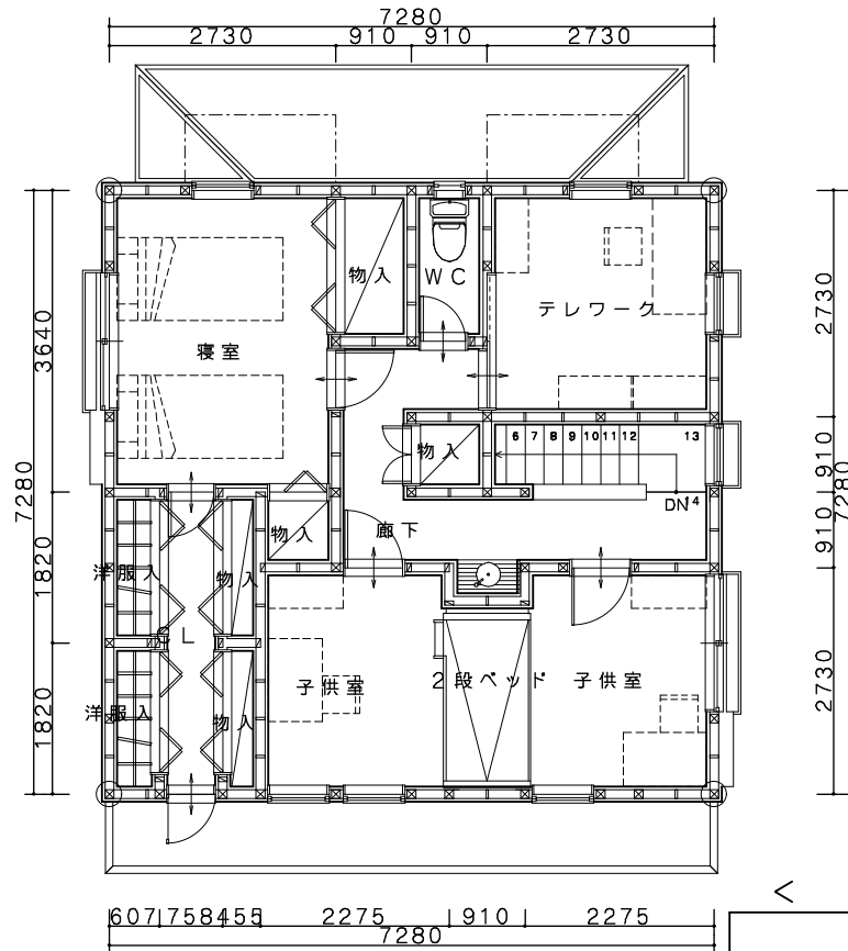
2階平面図
