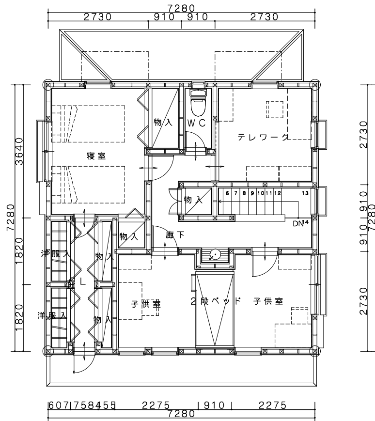
2階平面図
