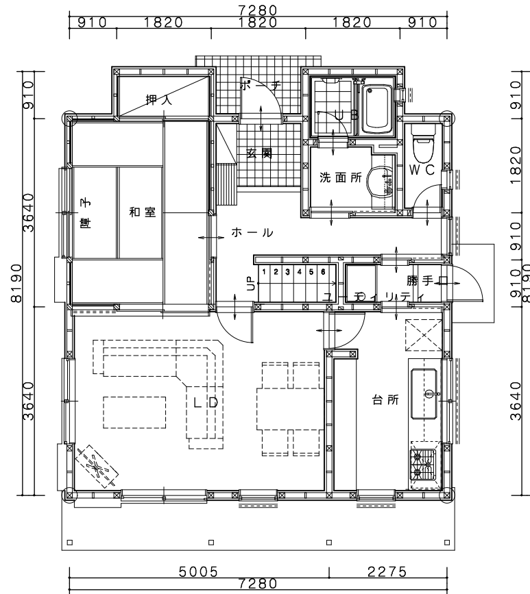
1階平面図
