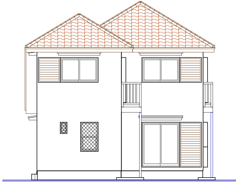
南側立面図
