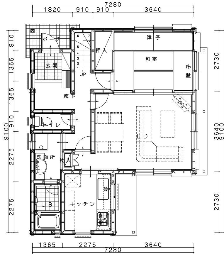
1階平面図
