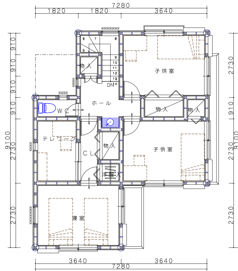
2階平面図
