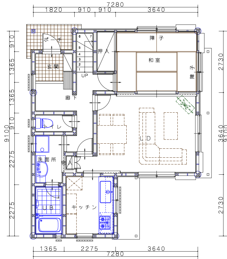
1階平面図
