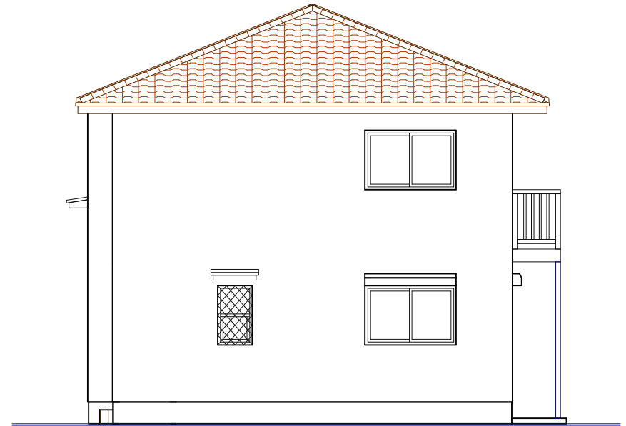
西側立面図
