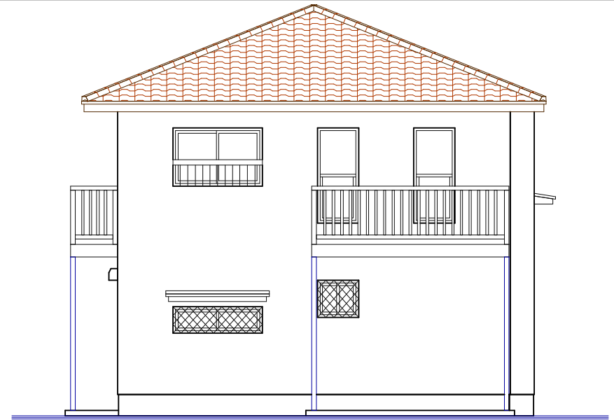
東側立面図
