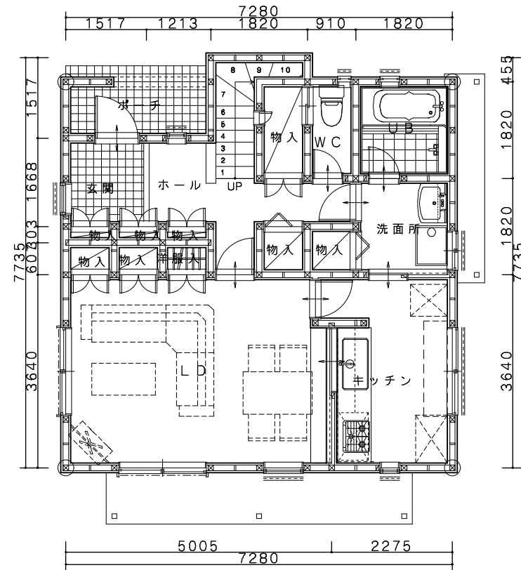
1階平面図
