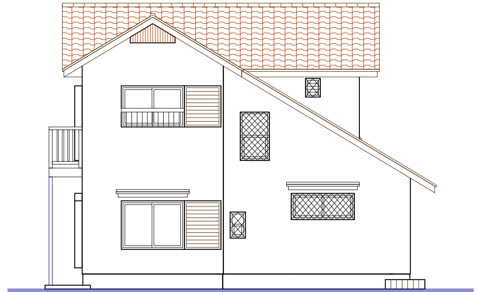
東側立面図
