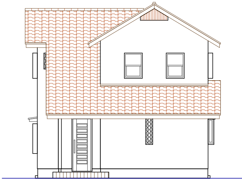
北側立面図
