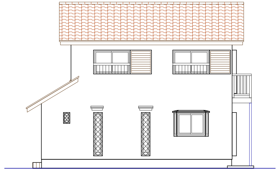
西側立面図
