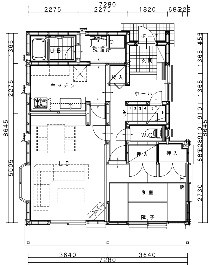
1階平面図
