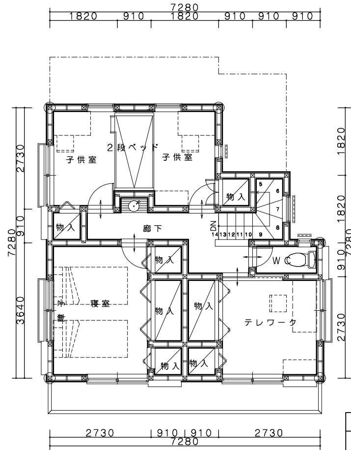
2階平面図
