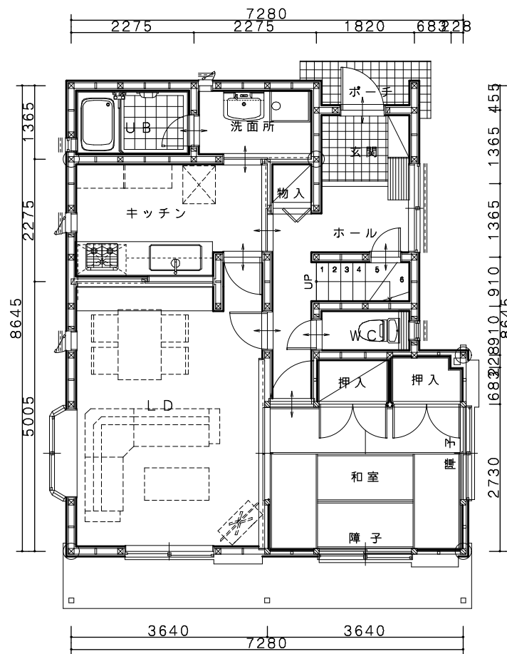
1階平面図
