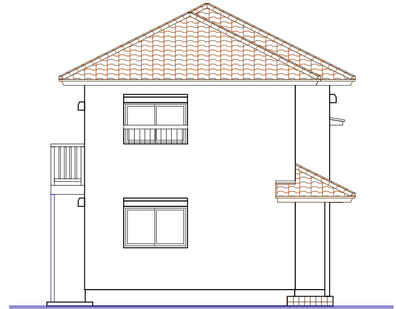
東側立面図
