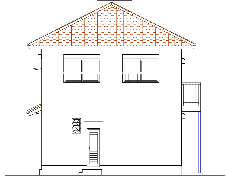
西側立面図
