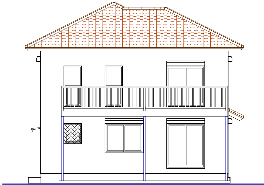
南側立面図
