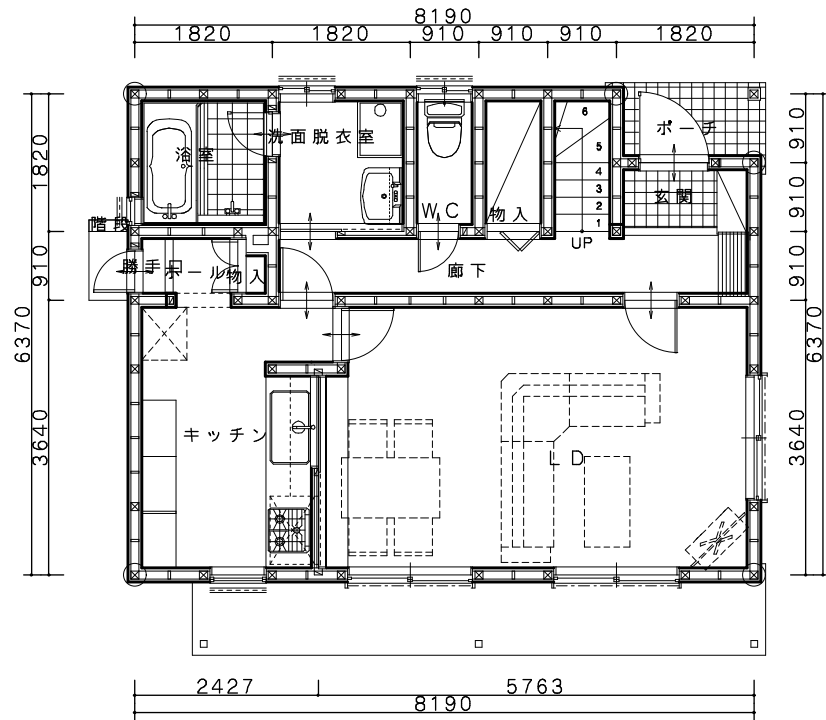
1階平面図
