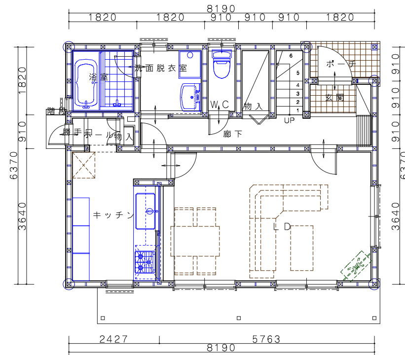
1階平面図
