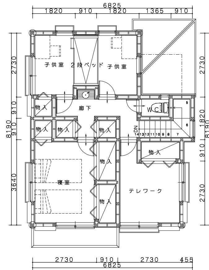
2階平面図
