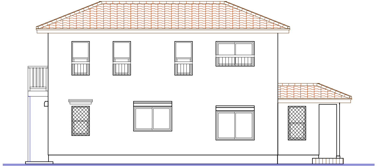
東側立面図
