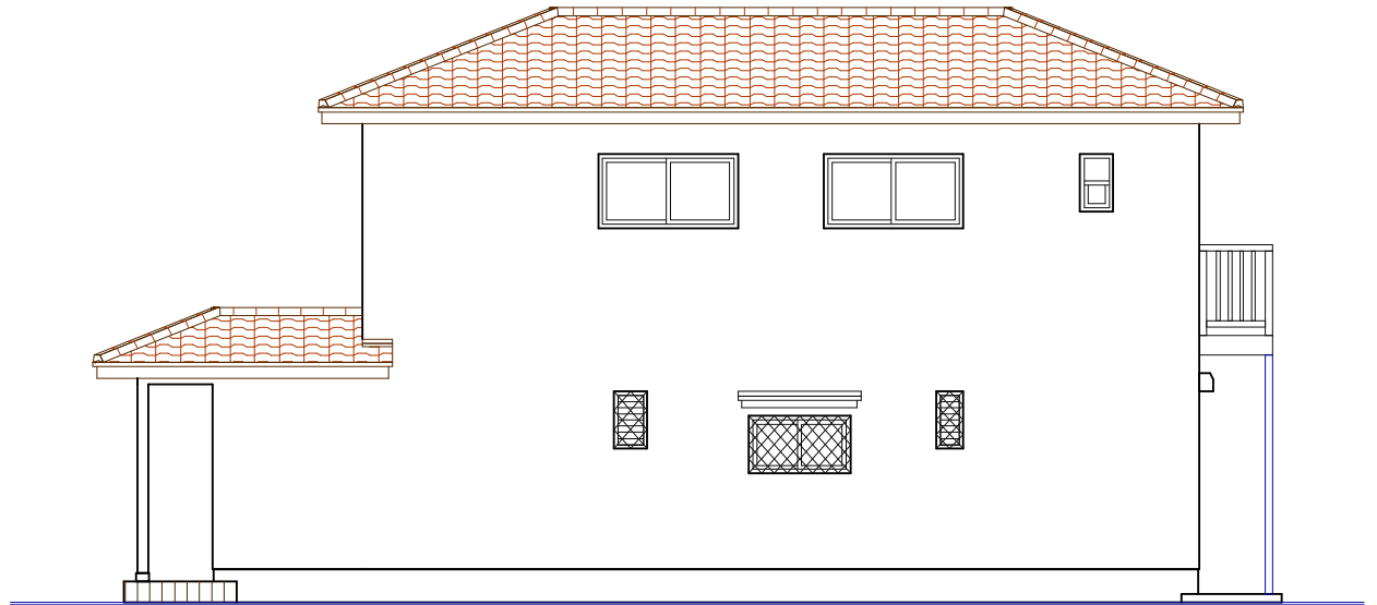
西側立面図
