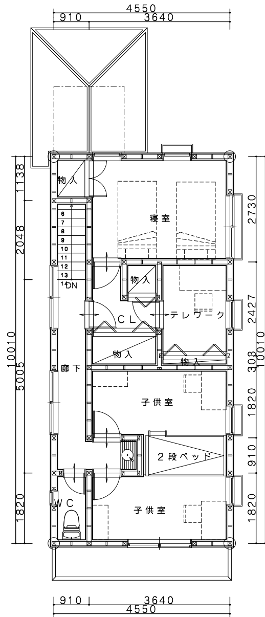
2階平面図
