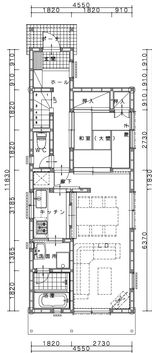
1階平面図
