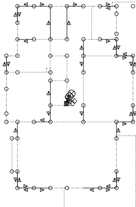
1階重心・剛心位置図 縮尺=1/100
