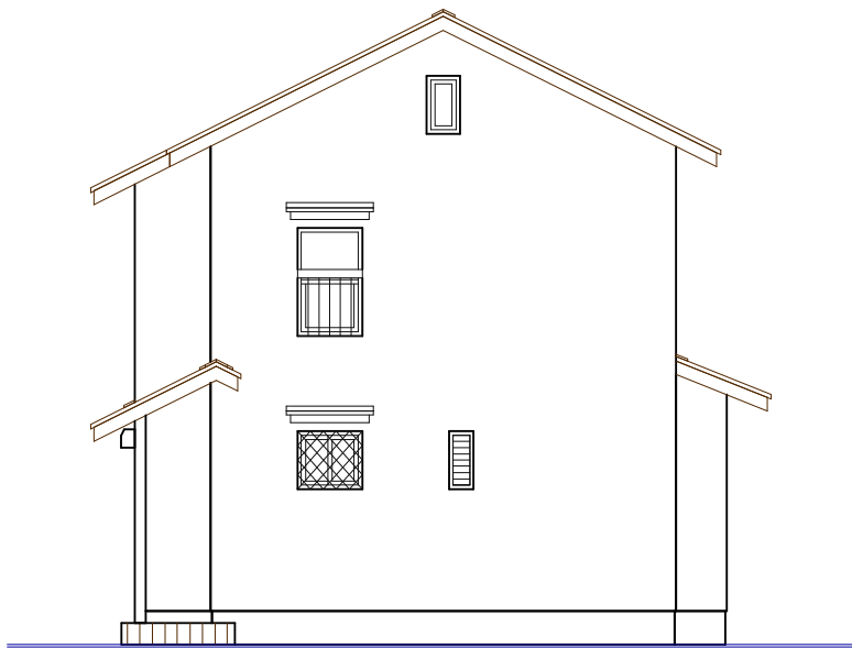
北側立面図
