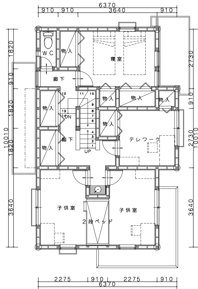
2階平面図
