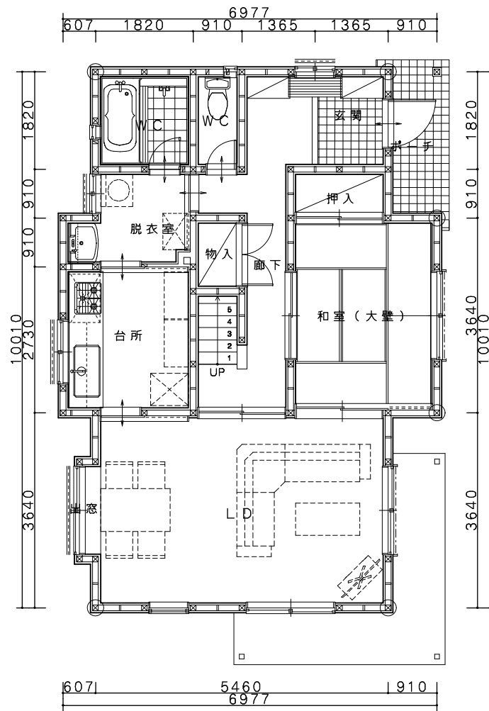
1階平面図
