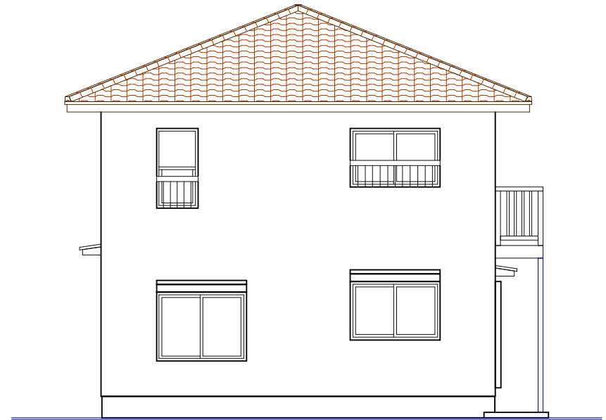
西側立面図
