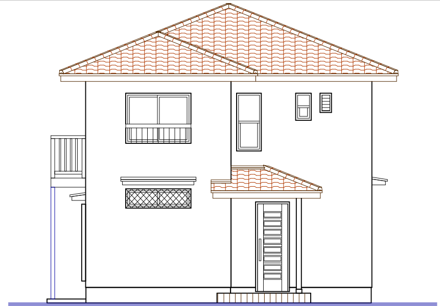
東側立面図
