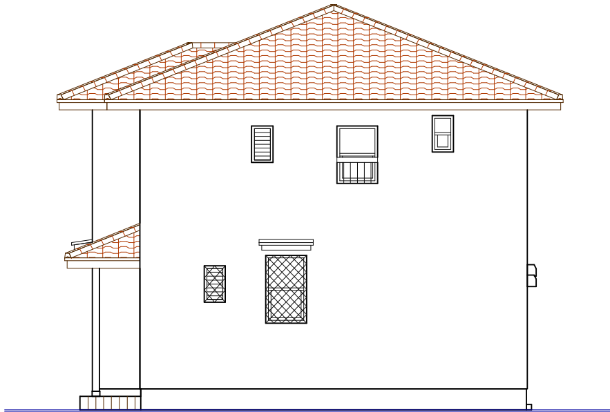
北側立面図
