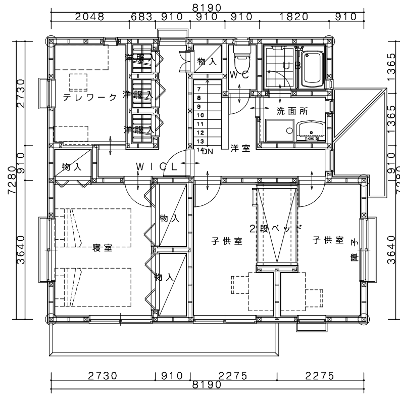
2階平面図
