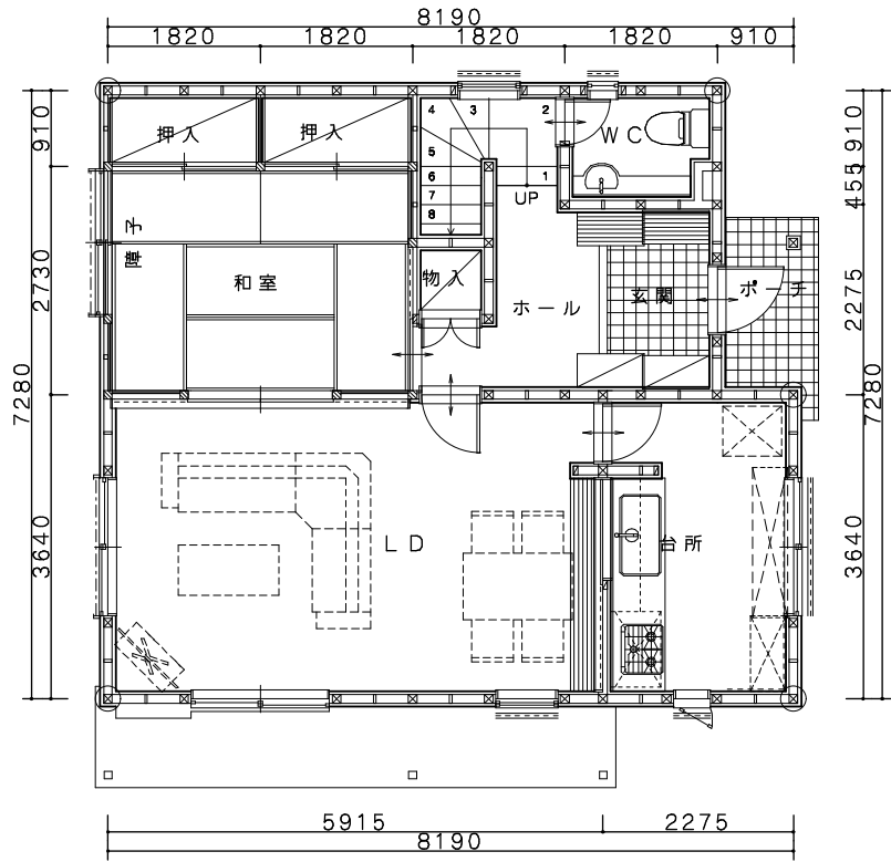
1階平面図
