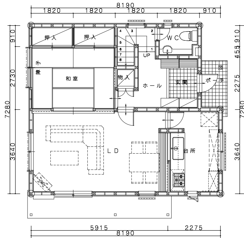
1階平面図
