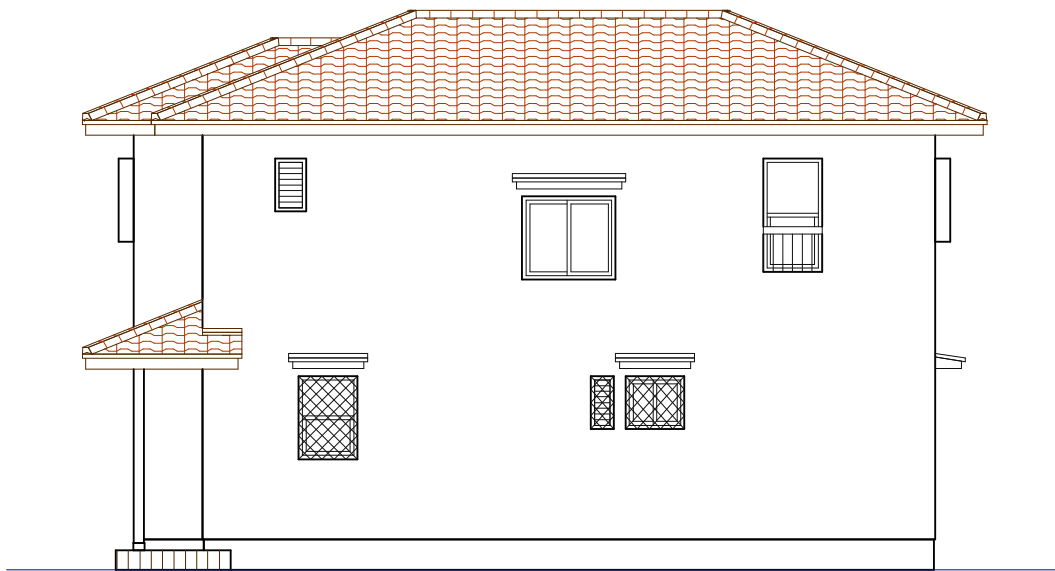
北側立面図
