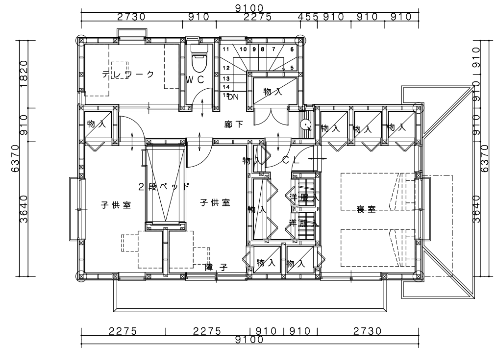
2階平面図
