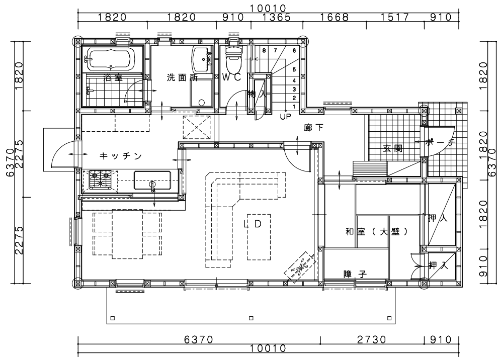
1階平面図
