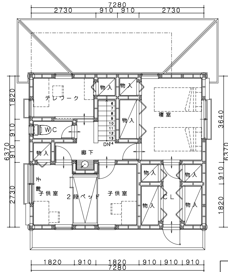
2階平面図
