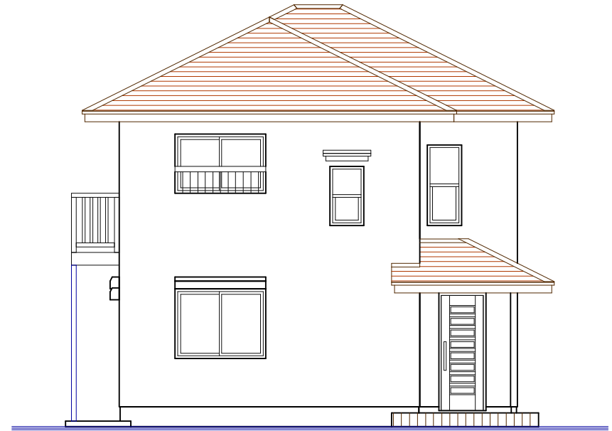
東側立面図
