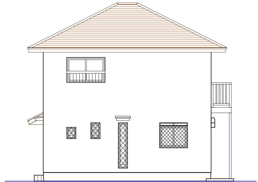
西側立面図
