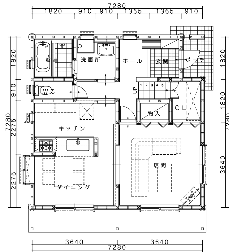
1階平面図
