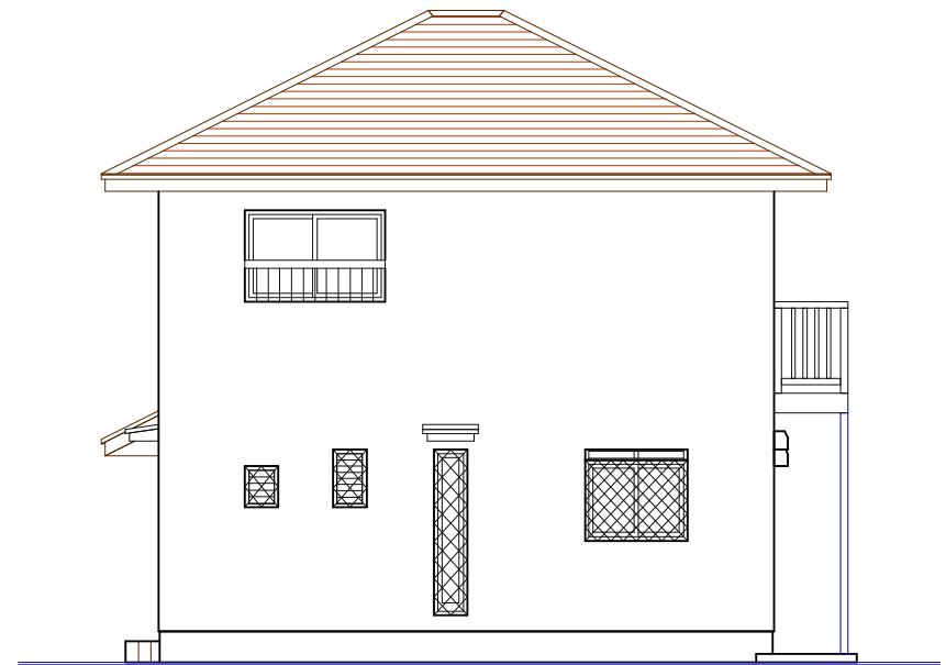
西側立面図
