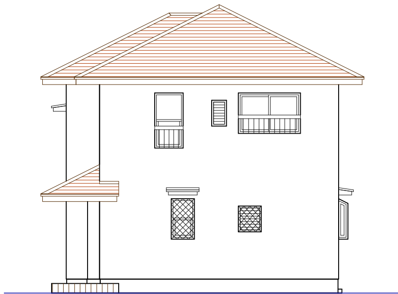
北側立面図
