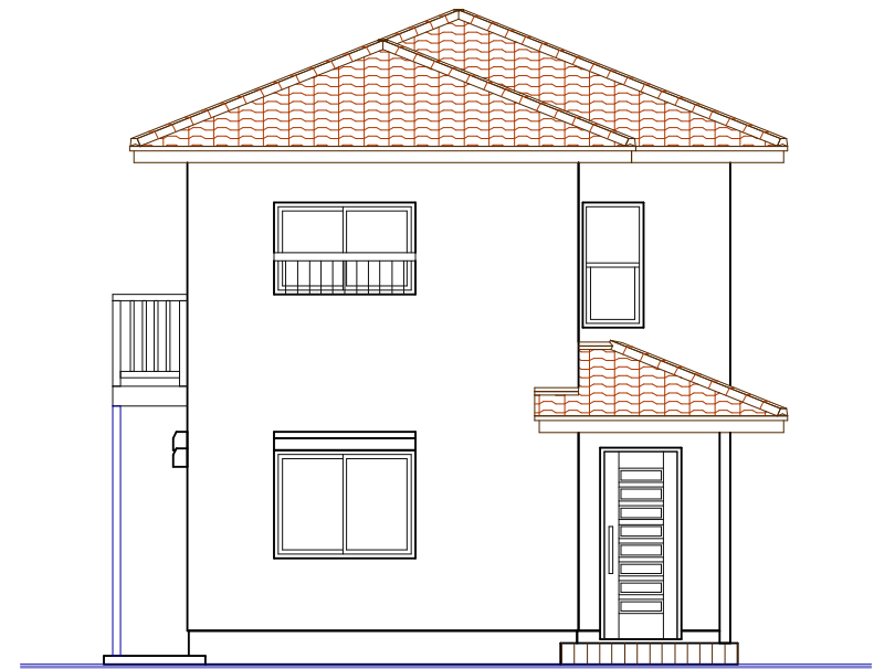
東側立面図
