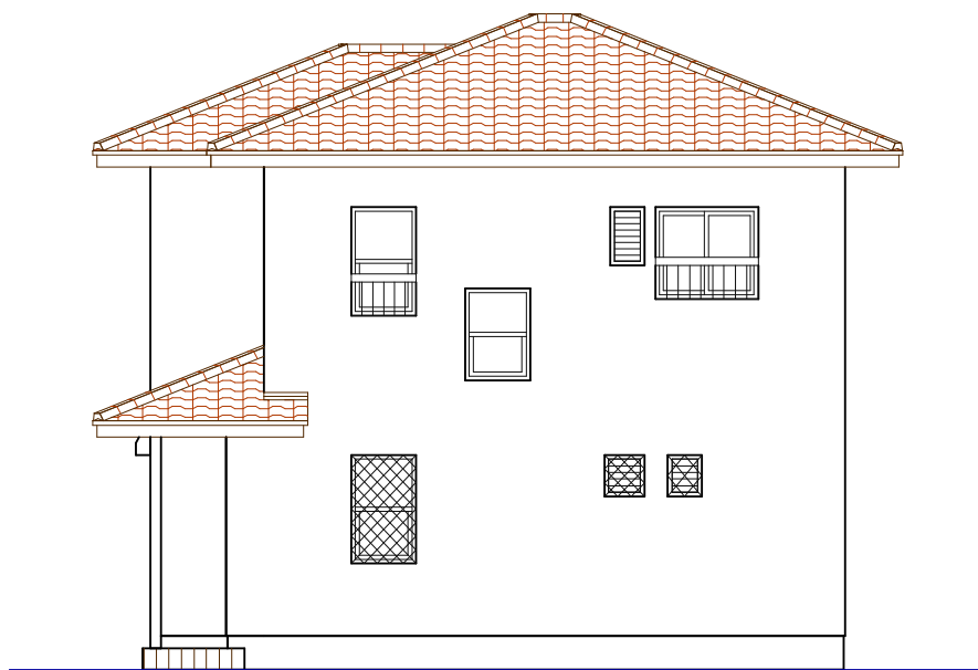
北側立面図
