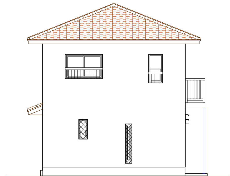
西側立面図
