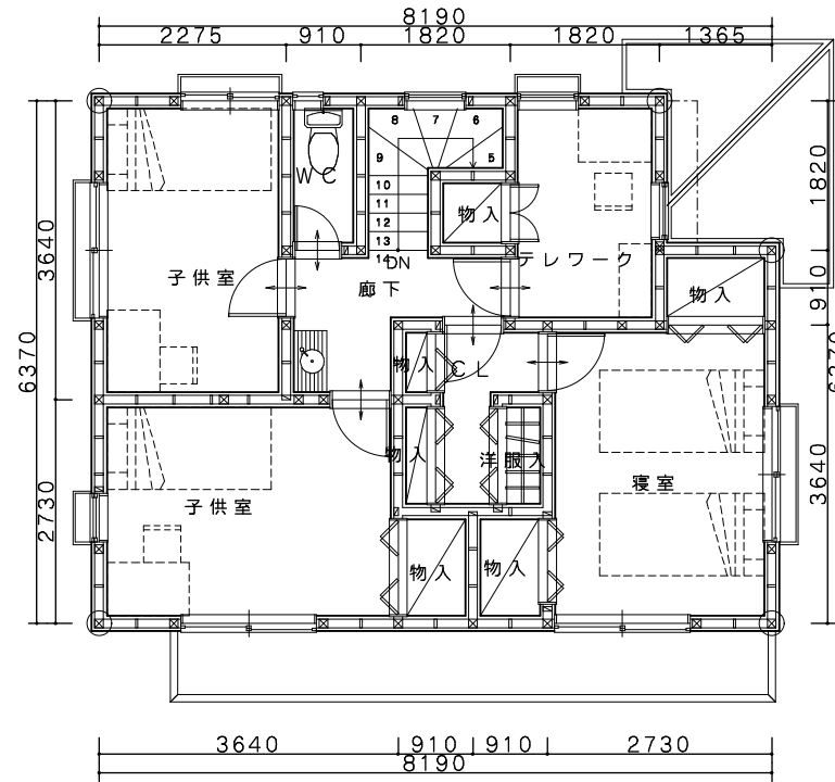
2階平面図
