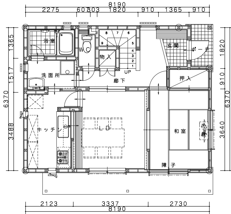
1階平面図
